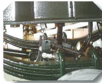
Suspension mécanique
